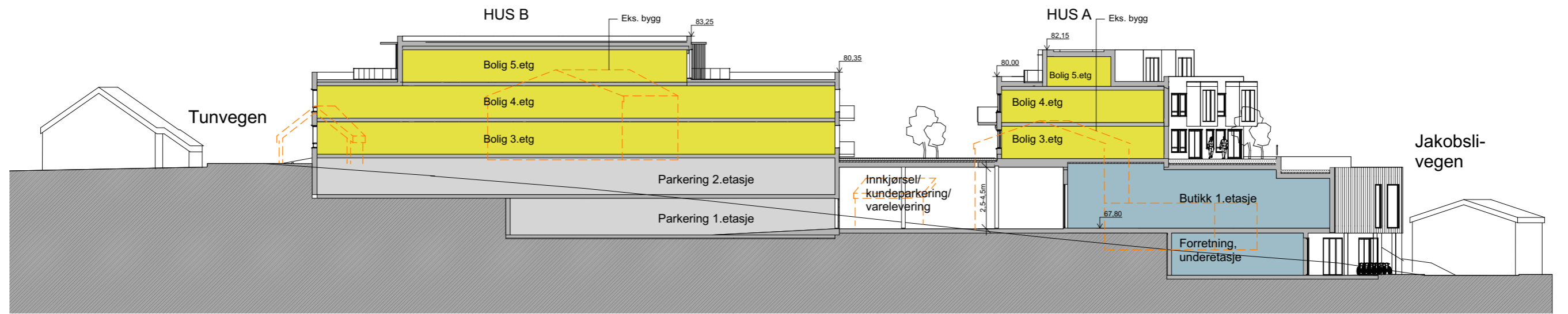
Snitt A
